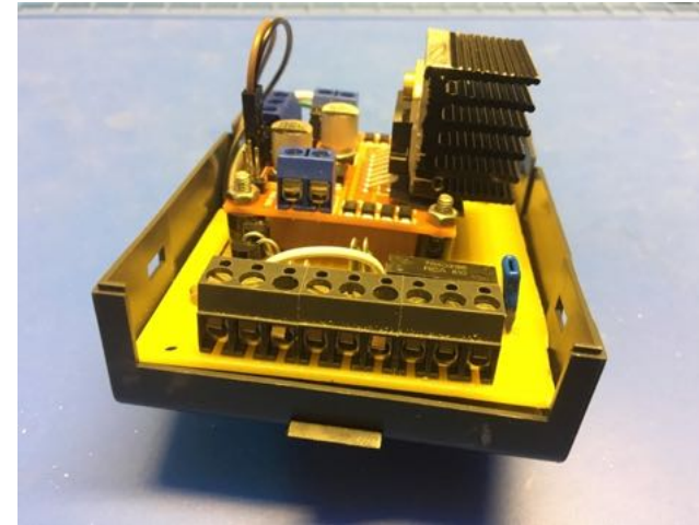
Größerer Kühlkörper in Strömungsrichtung
